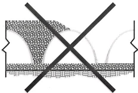
UNEVEN BACKFILL
