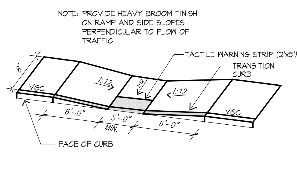
3 CURB CUT AND RAMP SCALE: N.T.S.
